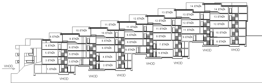
Prerez A-A M 1:1000
